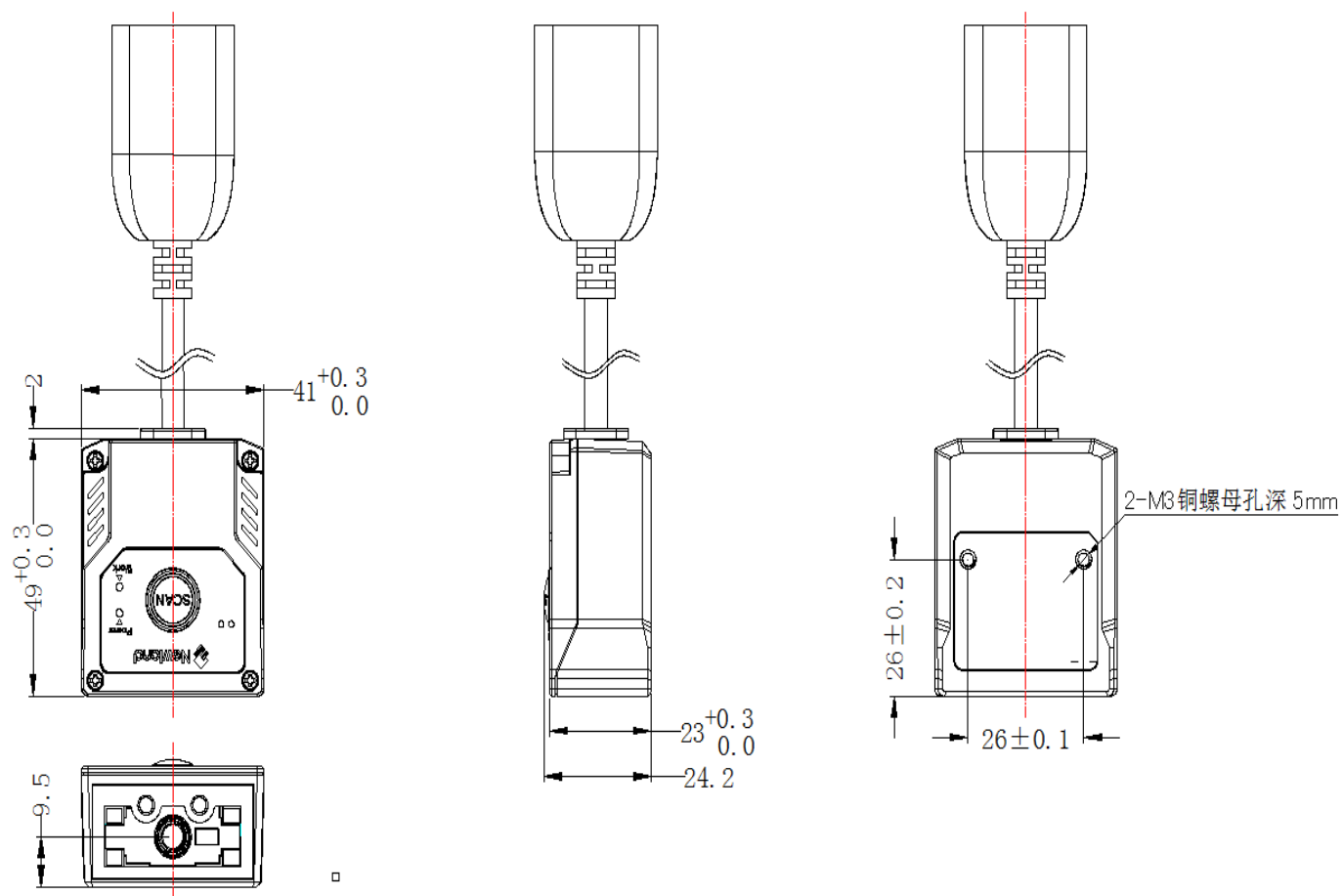
三视图
